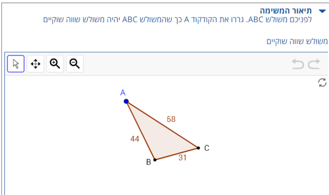
איור 1: היישומן.
